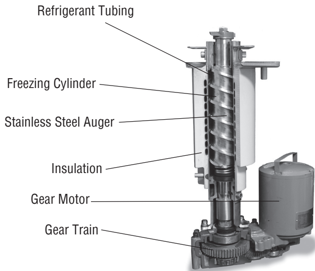
EVAPORATOR
